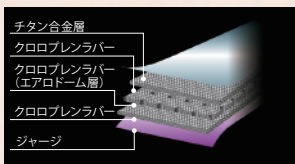
【エアロドーム構造図】
