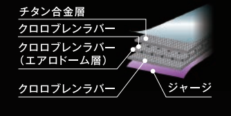
エアロドーム構造図
